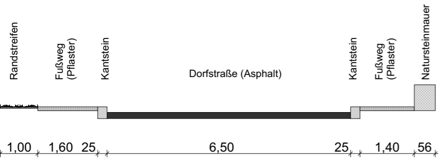
Schnitt Dorfstraße M. 1:100
