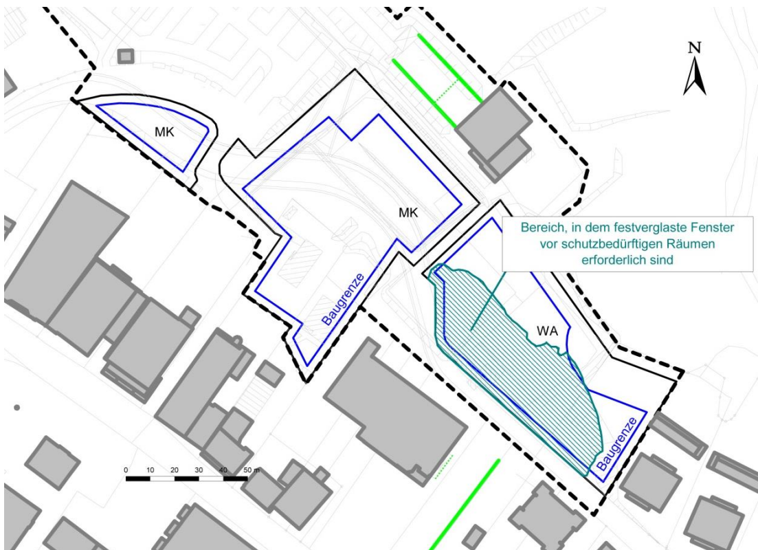
Darstellung der Bereiche zur Anordnung von schutzbedürftigen Räumen an der lärmabgewandten Gebäudeseite
