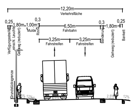
Planstraße B
