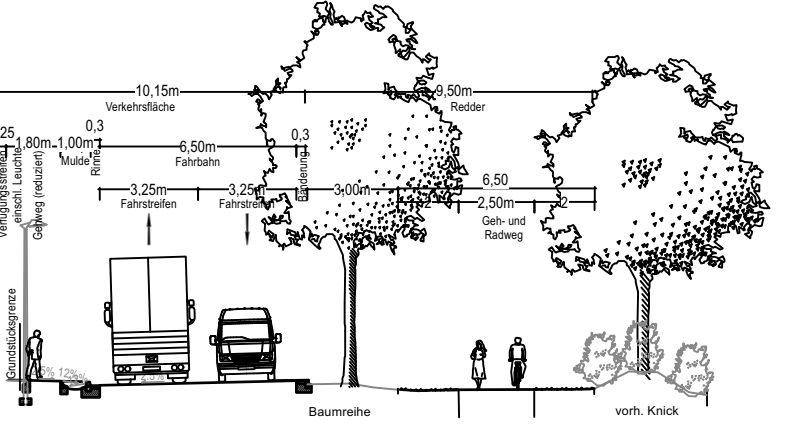
Planstraße C
