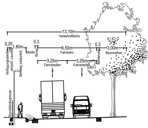
Planstraße A
