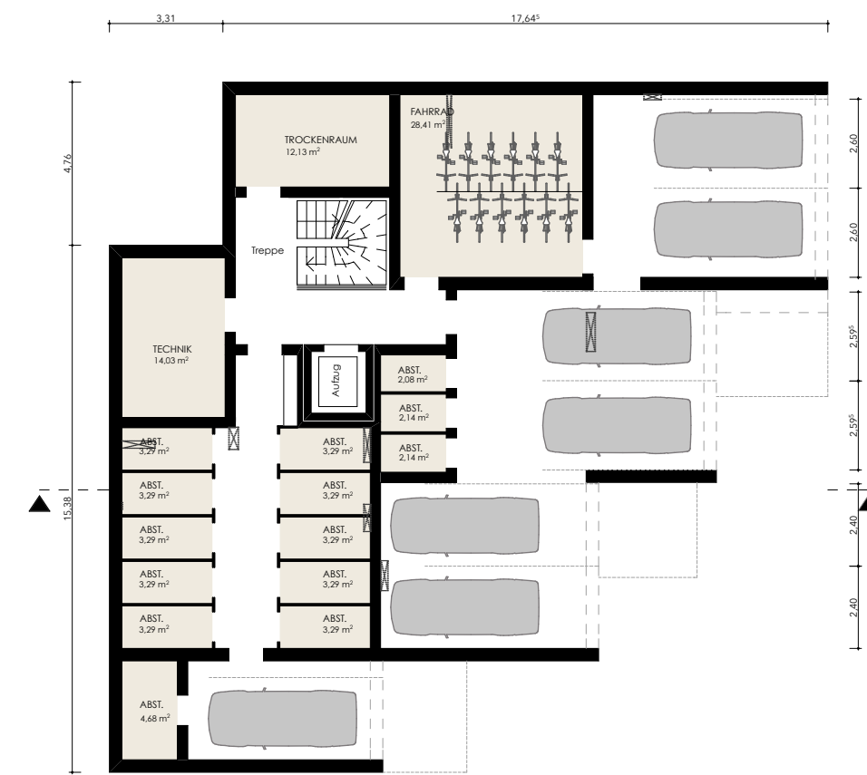
M 1_200 _ UNTERGESCHOSS
