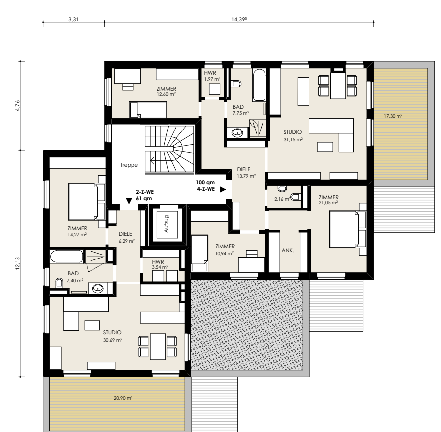
M 1_200 _ OBERGESCHOSS_2.2
