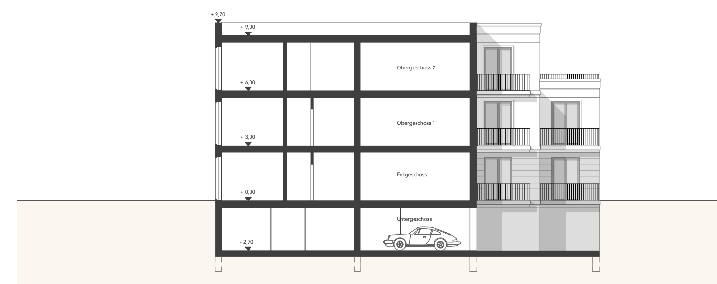
M 1_200 _ QUERSCHNITT
