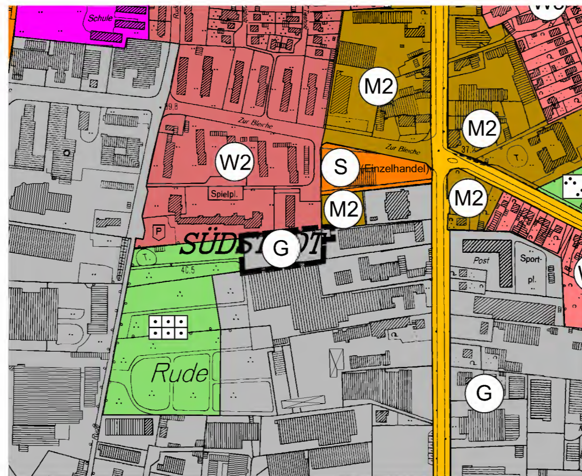
12. Berichtigung -Entwurf- Maßstab 1 : 5.000
