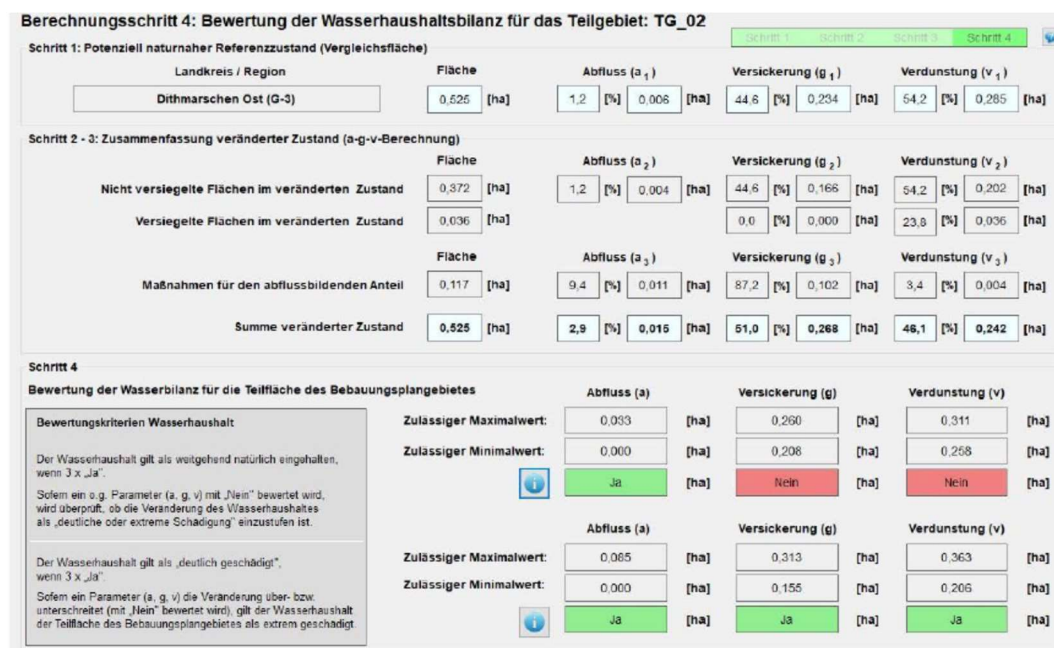
Abbildung 4: Berechnungsschritt 4 für Teilgebiet 2 aus dem Berechnungstool A-RW 1
