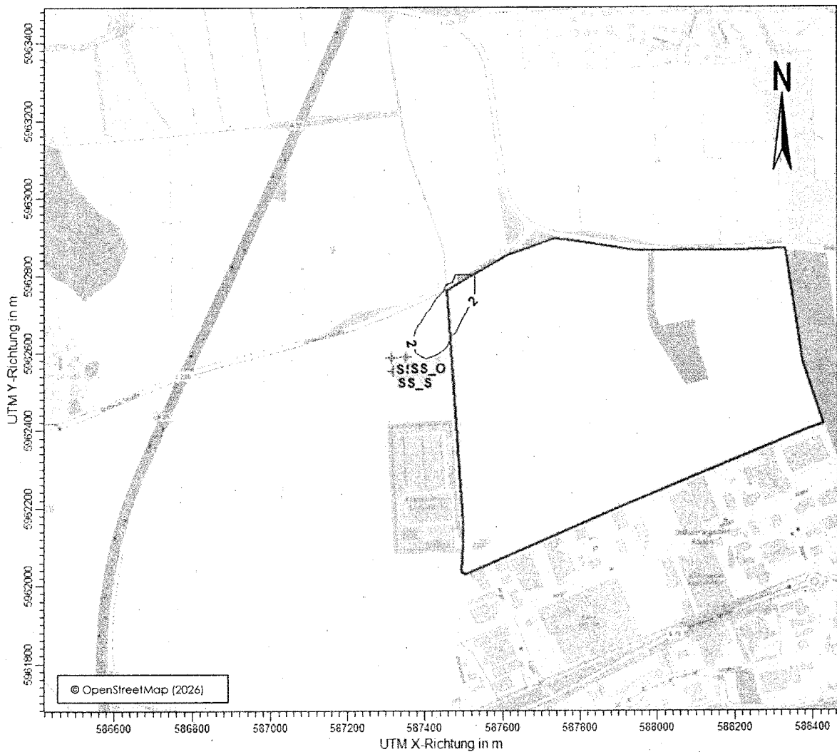
Abbildung 5: Gesamtzusatzbelastung IGZ durch den Betrieb der geplanten Heizzentrale in % der Jahresstunden, Isolinien-darstellung
