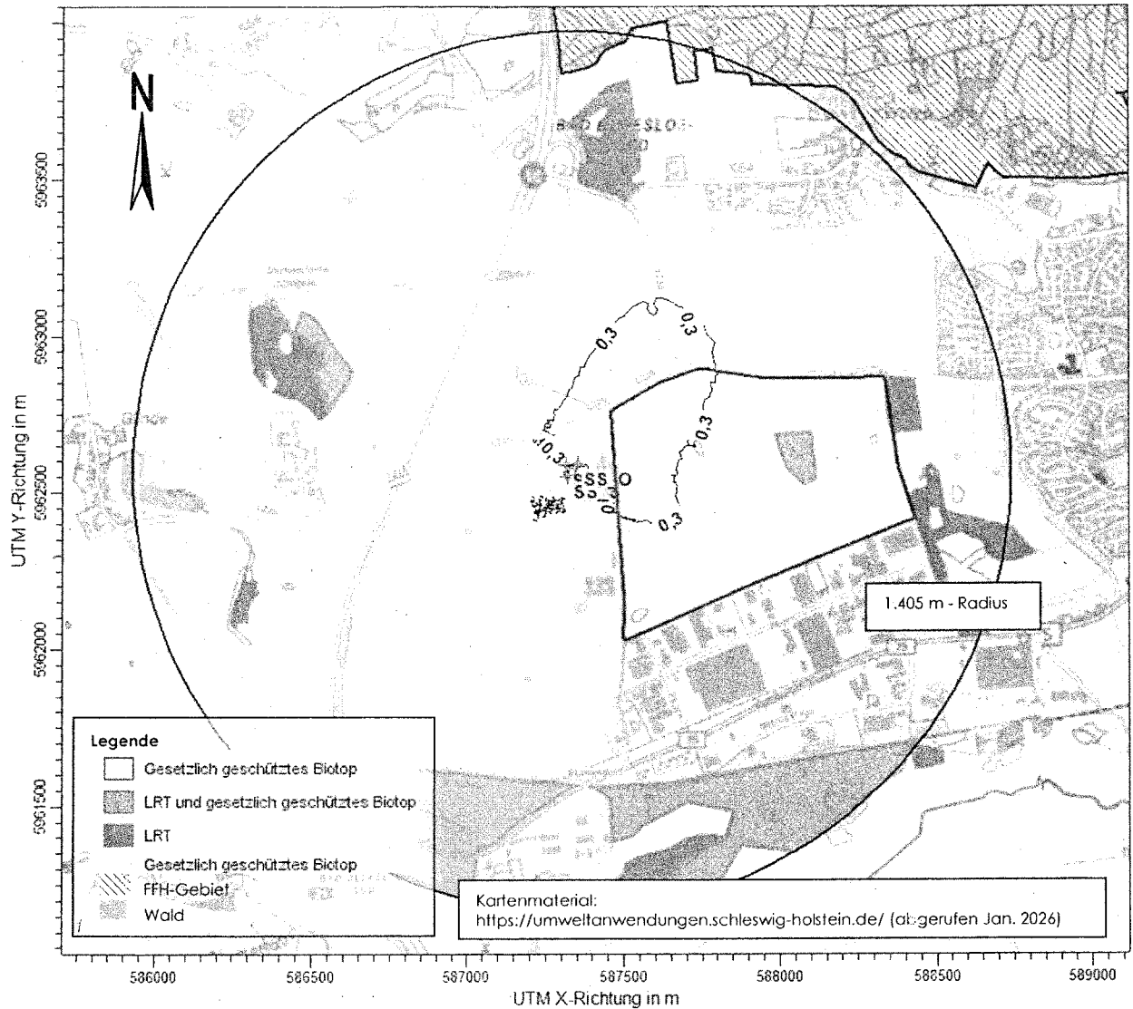
Abbildung 8: Stickstoffdeposition: Gesamtzusatzbelastung IGZ_{Plan} durch den Betrieb der geplanten Heizzentrale in \text{kg}/(\text{ha} \times \text{a}) , n(\text{meso})\text{-dep} (gültig für Mesoskala), Isolinien
