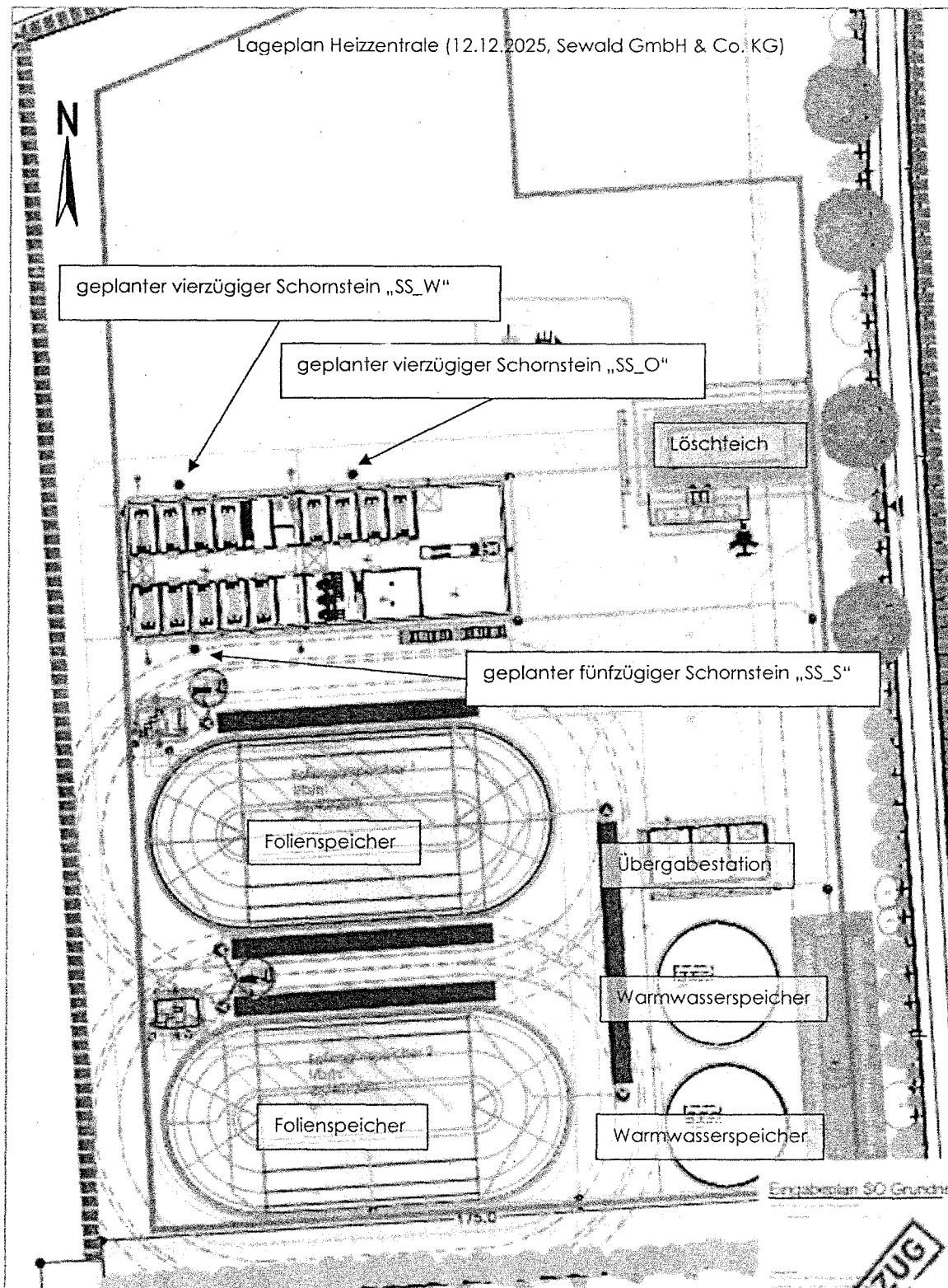
Abbildung 1: Auszug Lageplan
