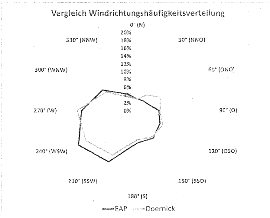
Abbildung 25: Vergleich Windrichtungsverteilung für EAP und Wetterstation Dörnack
