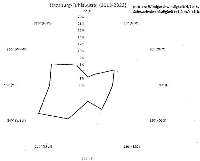
Abbildung 19: Windrichtungshäufigkeitsverteilung der Station Hamburg-Fuhlsbüttel
