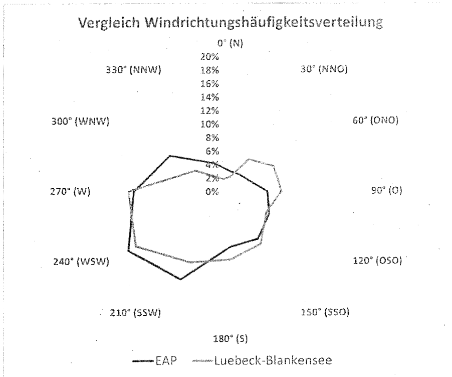
Abbildung 22: Vergleich Windrichtungsverteilung für EAP und Wetterstation Lübeck-Blankensee
