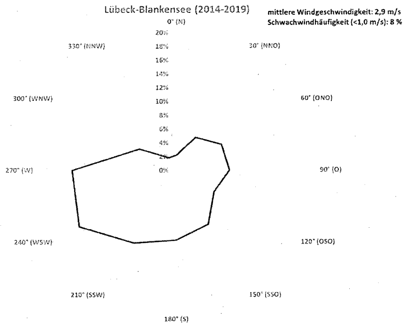
Abbildung 18: Windrichtungshäufigkeitsverteilung der Station Lübeck-Blankensee
