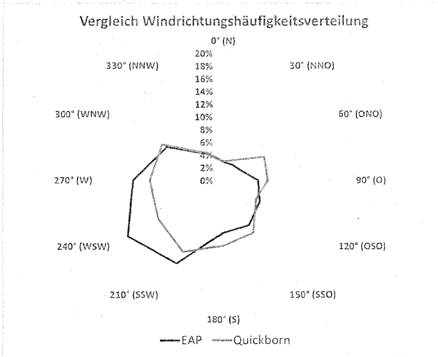
Abbildung 24: Vergleich Windrichtungsverteilung für EAP und Wetterstation Quickborn
