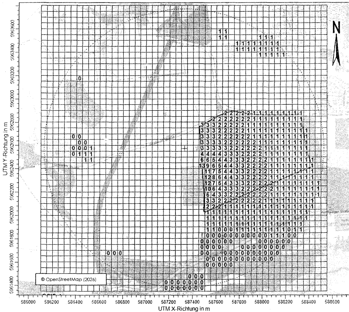
Abbildung 7: Gesamtbelastung IG durch die geplante Heizzentrale und die BGA in geändertem Zustand in % der Jahressstunden, Seitenlänge: 50 m
