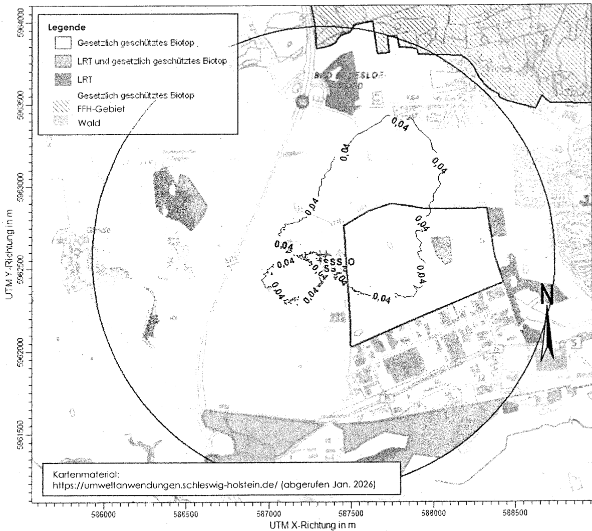
Abbildung 11: Säure: Gesamtzusatzbelastung IG ZPlan durch den Betrieb der geplanten Heizzentrale in \text{kg}/(\text{ha} \times \text{a}) für Wald, a(\text{wald}) (gültig für Wald)
