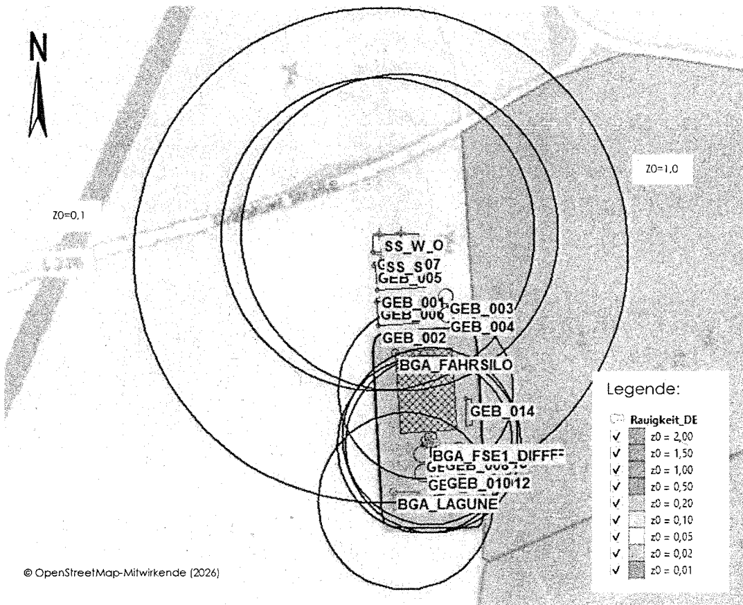
Abbildung 26: Grafische Darstellung der Rauigkeitslängen
