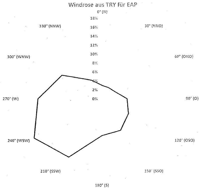
Abbildung 16: Windrichtungshäufigkeitsverteilung TRY-Daten für den EAP-Standort
