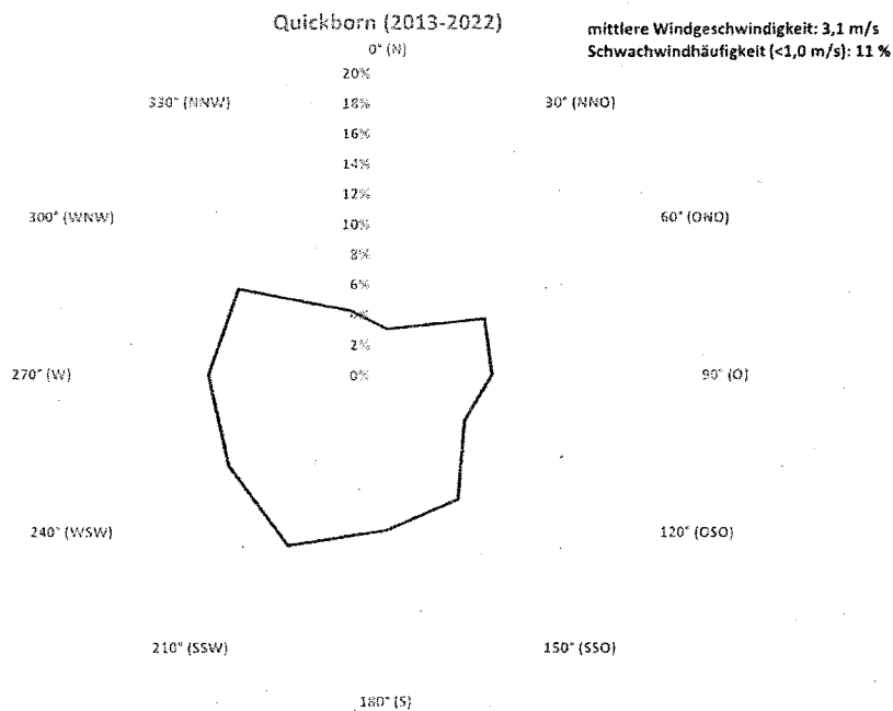
Abbildung 20: Windrichtungshäufigkeitsverteilung der Station Quickborn
