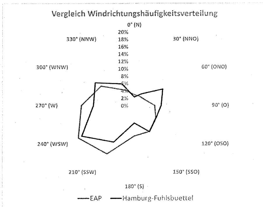
Abbildung 23: Vergleich Windrichtungsverteilung für EAP und Wetterstation Hamburg-Fuhlsbüttel
