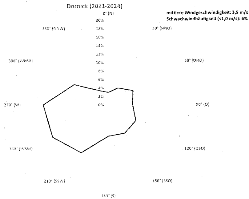
Abbildung 21: Windrichtungshäufigkeitsverteilung der Station Dörnick
