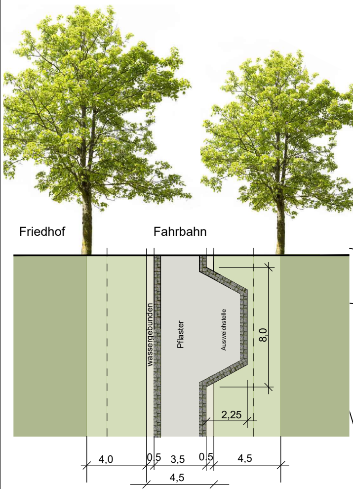
Schematischer Straßenquerschnitt
