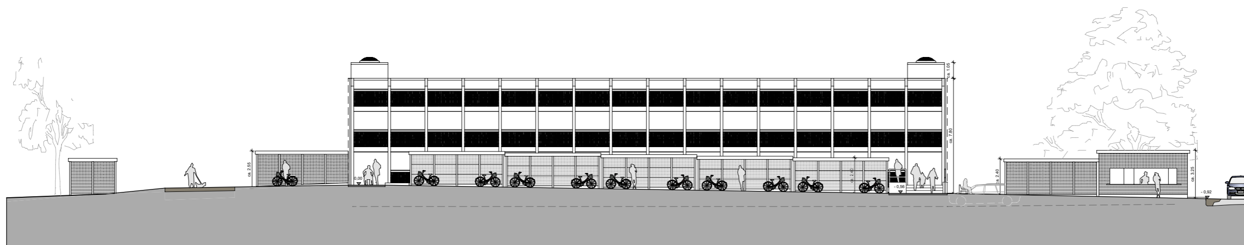
Ansicht B-B Heidkampstraße
