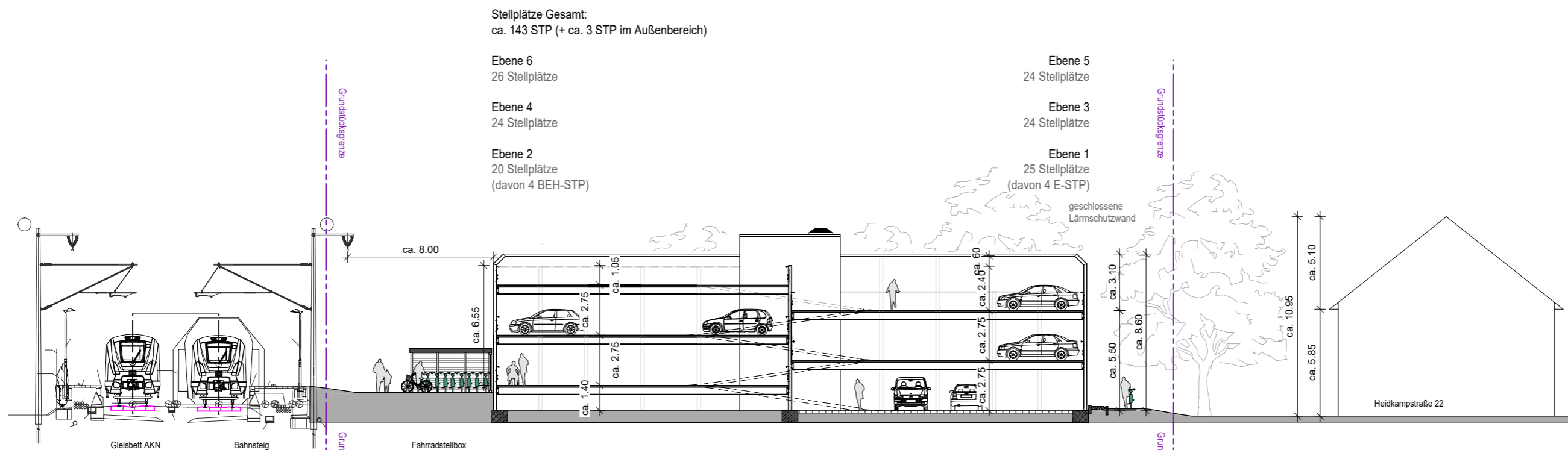
Schnitt A-A
