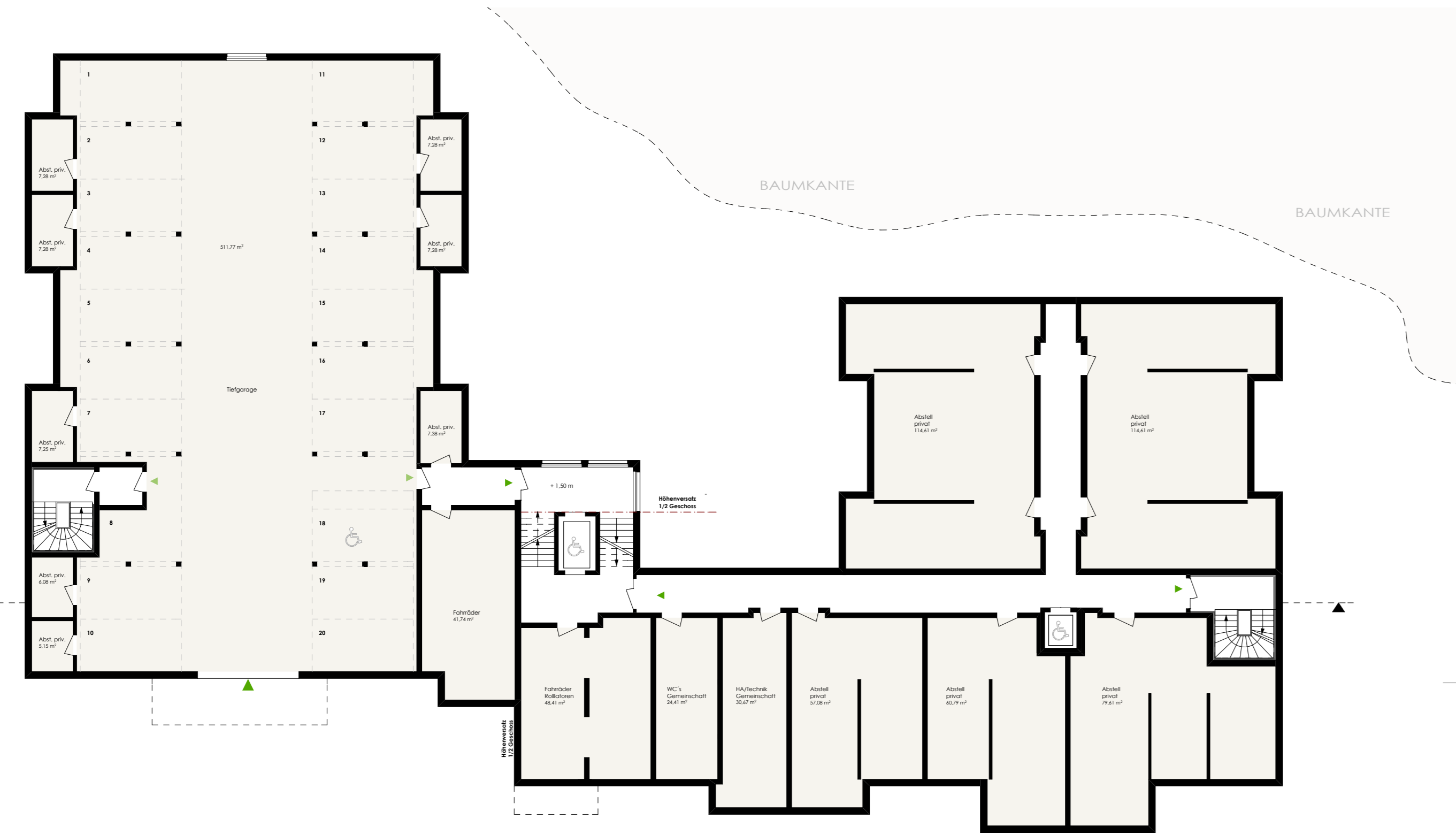
M 1,200 _ UNTERGESCHOSS
