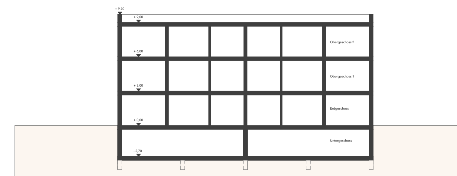
M 1_200 _QUERSCHNITT
