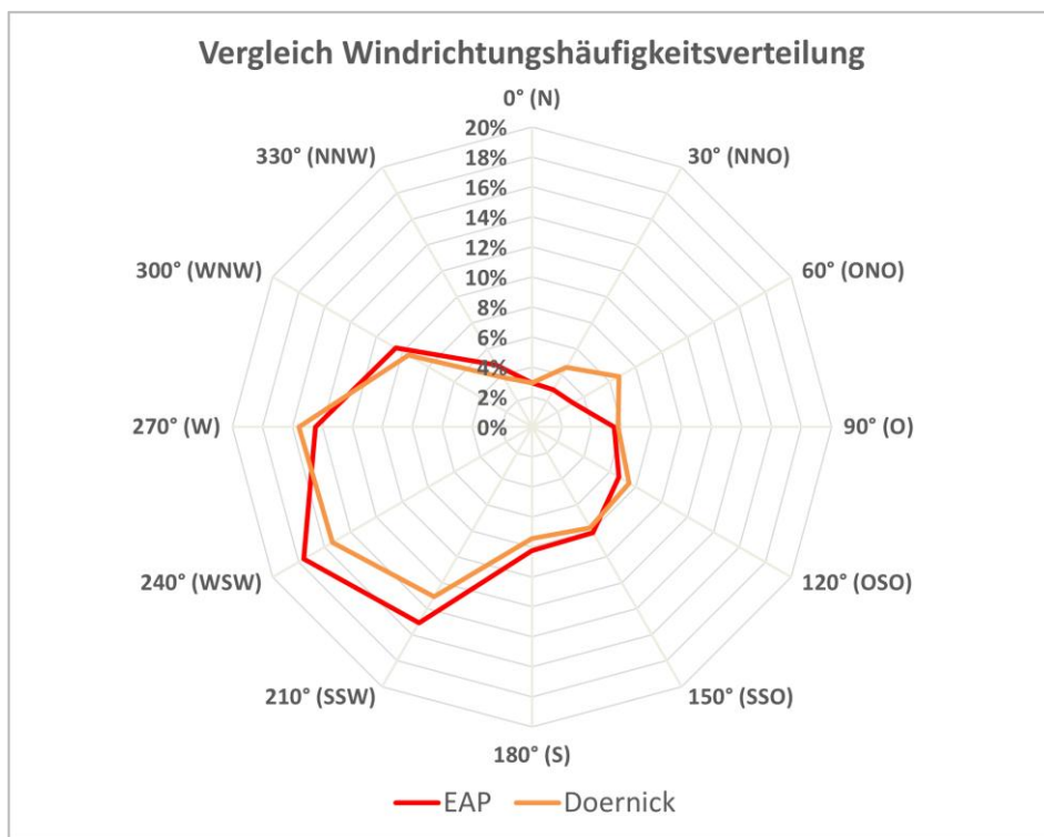
Abbildung 25: Vergleich Windrichtungsverteilung für EAP und Wetterstation Dörnack
