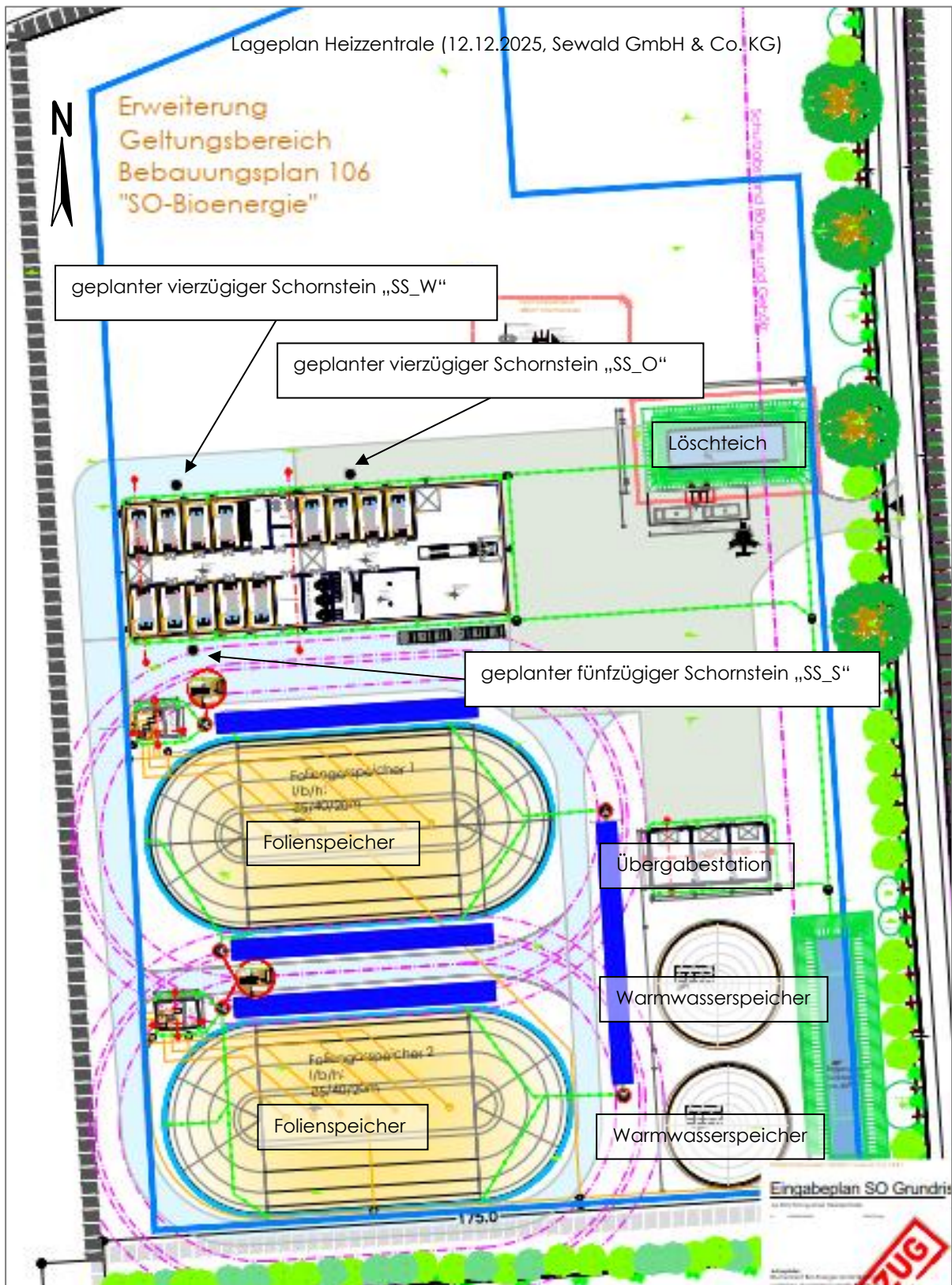
Abbildung 1: Auszug Lageplan
