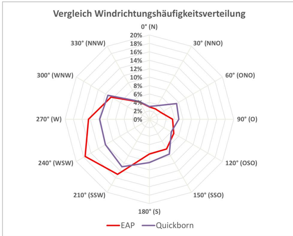
Abbildung 24: Vergleich Windrichtungsverteilung für EAP und Wetterstation Quickborn
