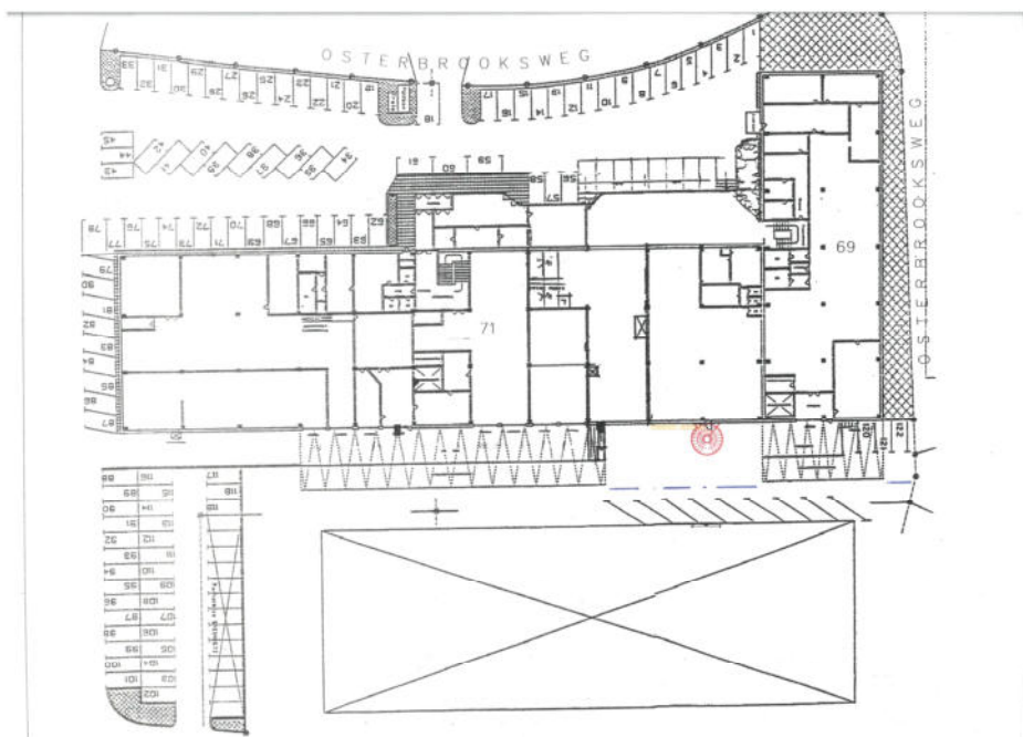
Abbildung 15 – System-Grundriss mit vierachsigem (multifunktionalem) Stützenraster
