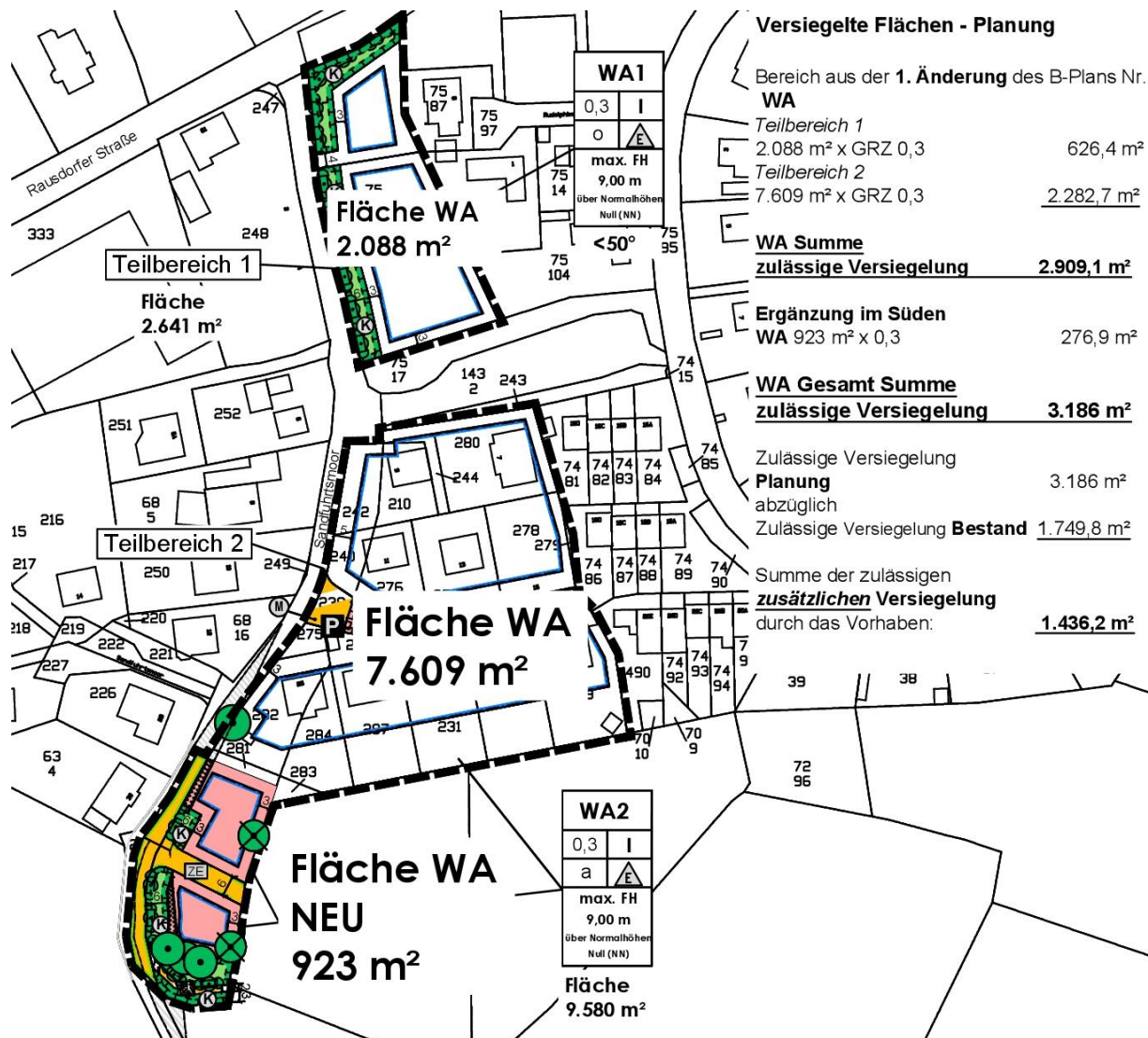
Abbildung 23: Darstellung der zulässigen versiegelten Flächen in der Planung
