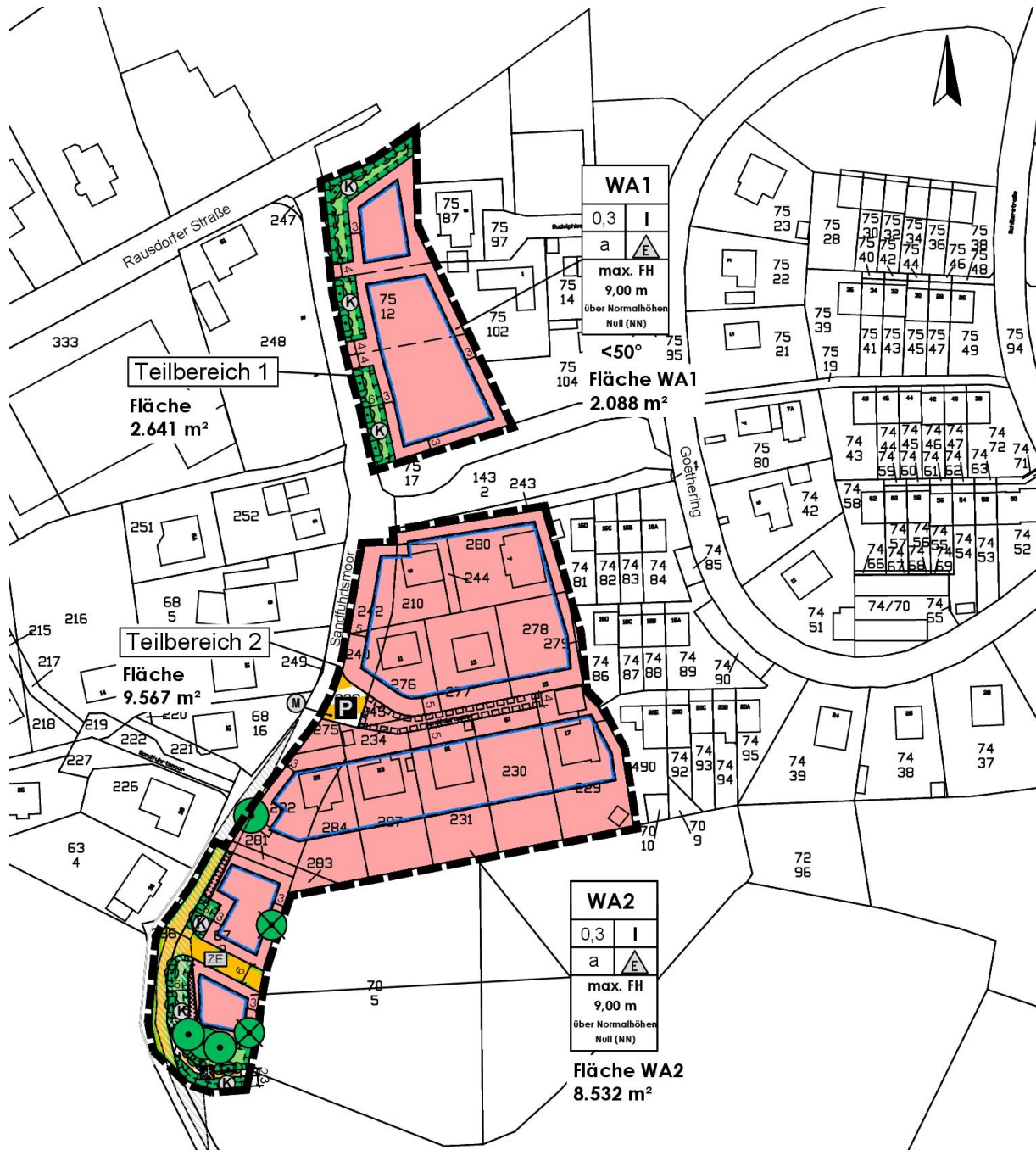
Abbildung 20: Auszug aus der Planzeichnung
