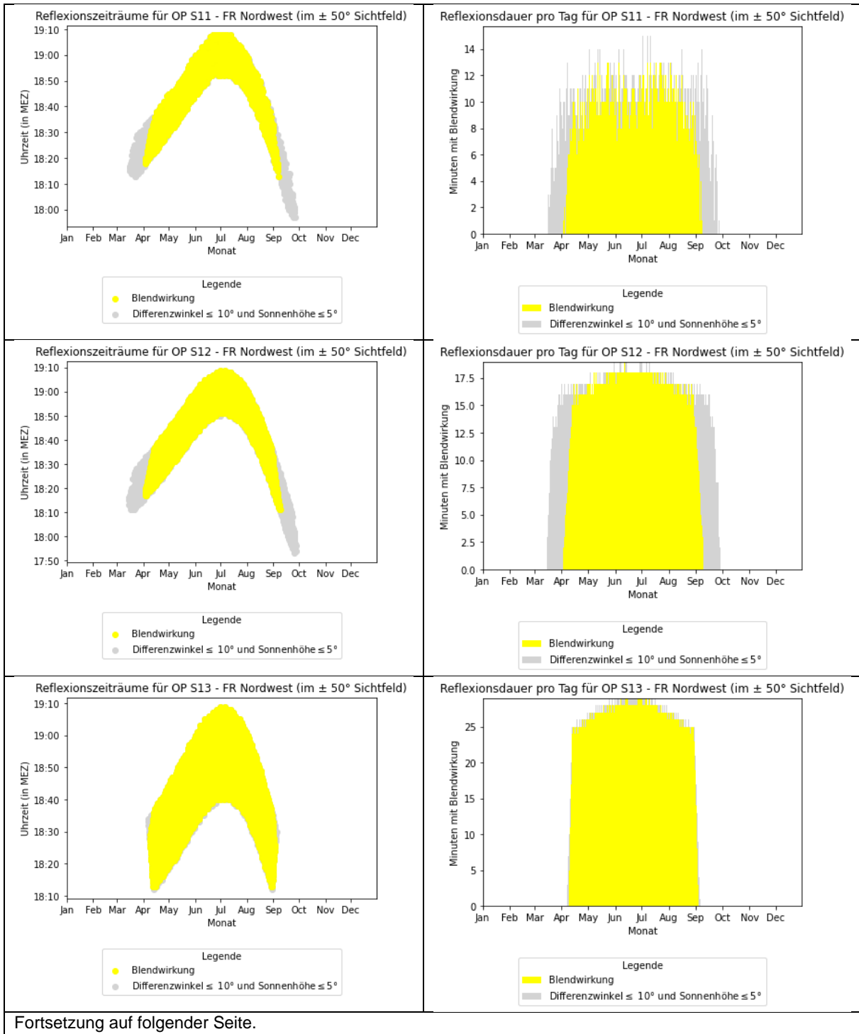
Ergebnisdiagramme 1: Relevante Reflexionen auf die Verkehrswege, welche innerhalb der Erheblichkeitsgrenze ( \pm 50^\circ Sichtfeld) wahrgenommen werden können
