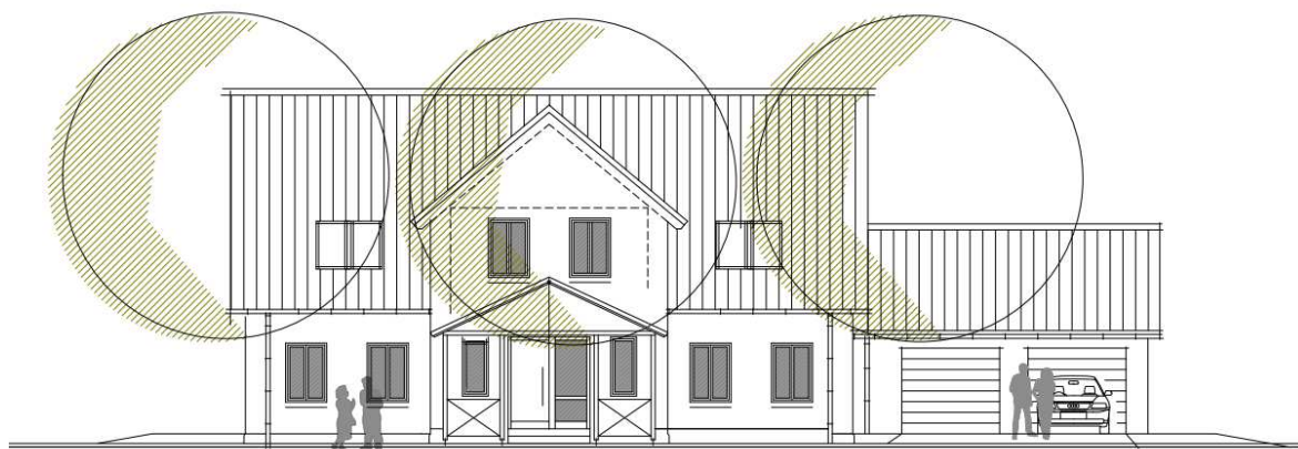
Abb. 12: Vorentwurf Einfamilienhaus
